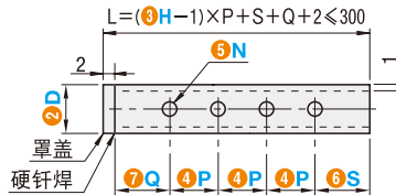
直管型
