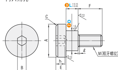
内六角孔
