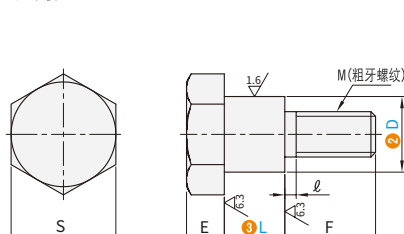
六角头型
