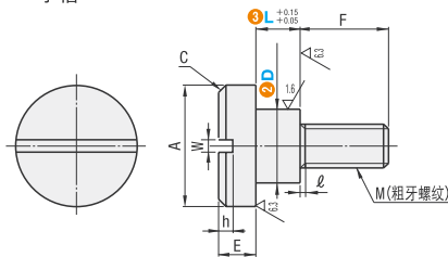
一字槽
