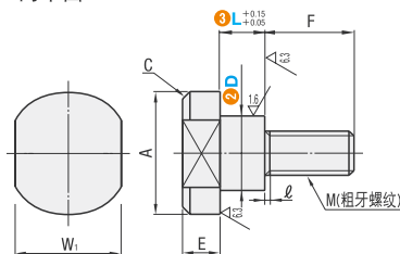
两平面
