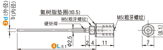
(外螺纹·内螺纹型) (高度调整用外螺纹·内螺纹型)
