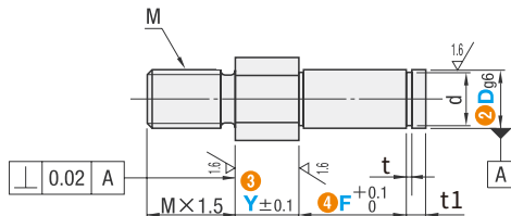
螺纹长度固定型
