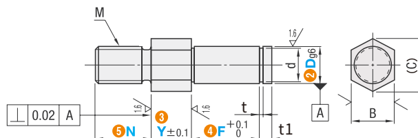
螺纹长度指定型
