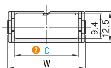
外径开口
